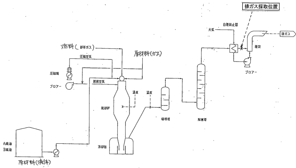
図-1 排ガス採取位置
